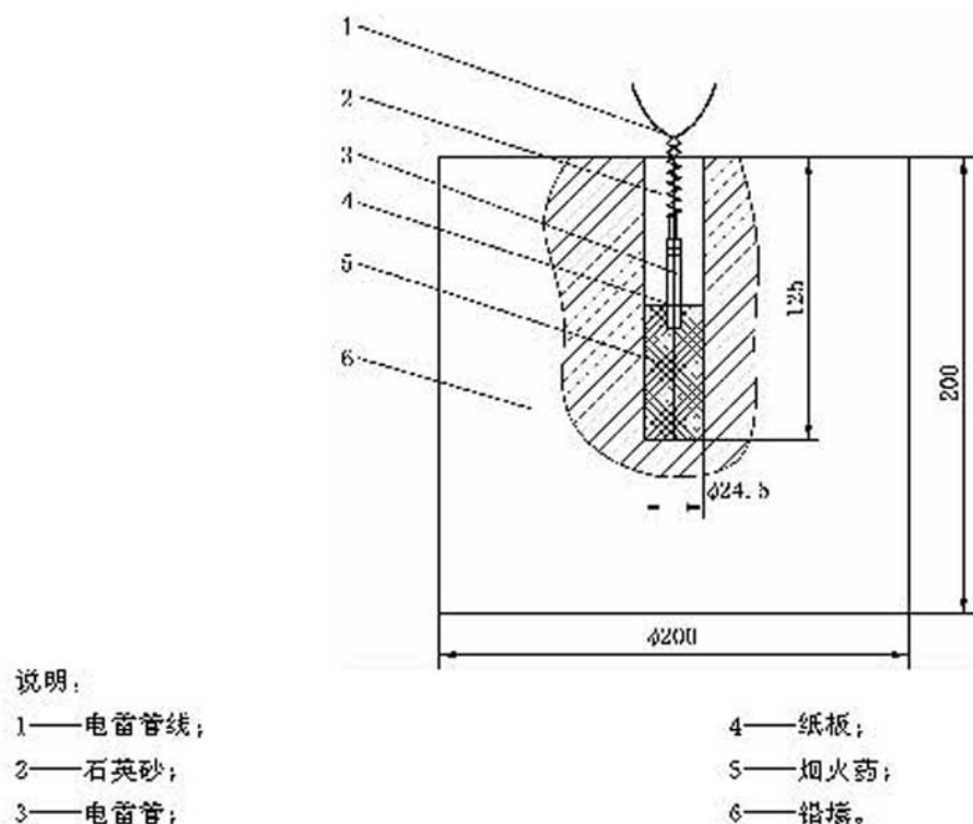
图 3 爆炸扩张铅罐中心孔装置示意图
